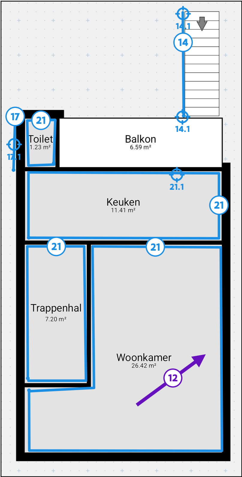
Legende van plan 1.6: Eerste verdieping
